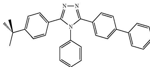
NTAZ
