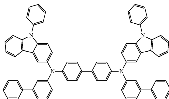
HT20
