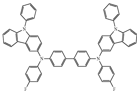
HT16
